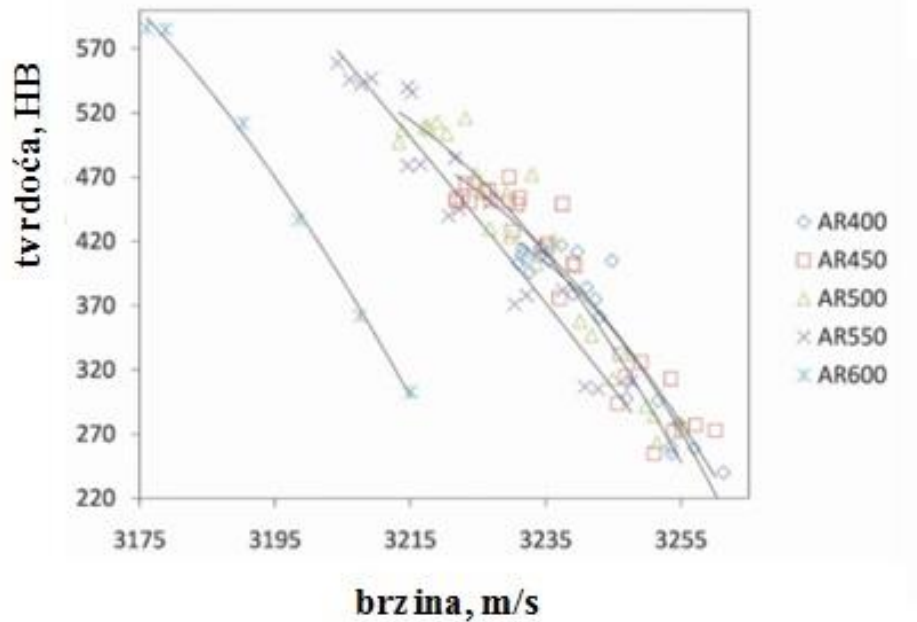
Slika 10. Korelacija tvrdoće i izračunate brzine T valova [2]
