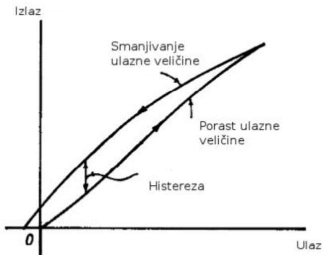
Slika 15. Histereza.
