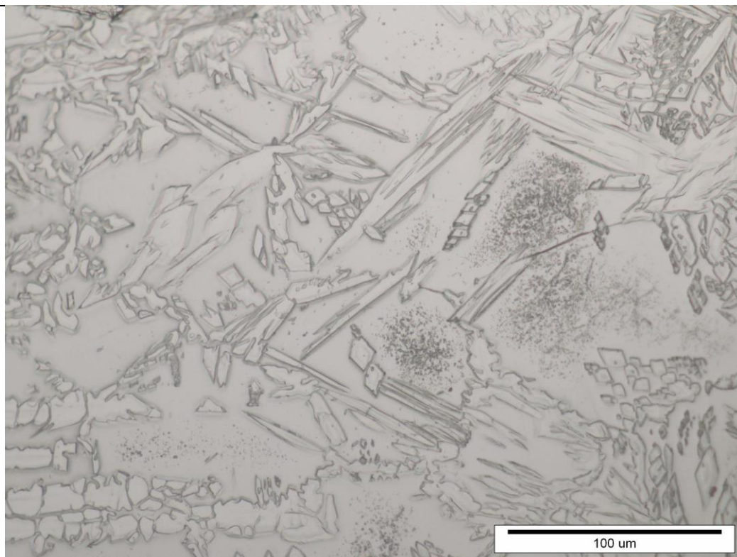
Slika 37. Mikrostruktura u tjemenu ZUT-a lijevo, snimljena pri povećanju od 500 puta
