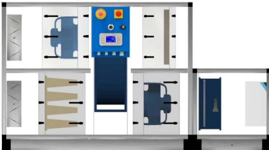
Slika 24: Klima komora za pripremu zraka
