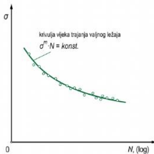
Slika 7. Krivulja vijeka trajanja valjnog ležaja [2]
