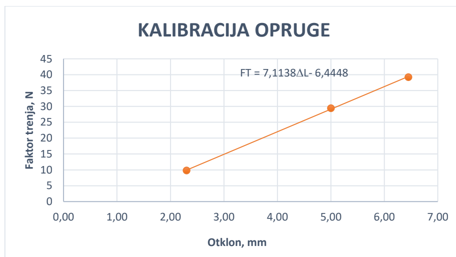
Slika 30. Kalibracija opruge za ispitivanje otpornosti na adhezijsko trošenje polaznog prstena i nitiranog u plazmi
