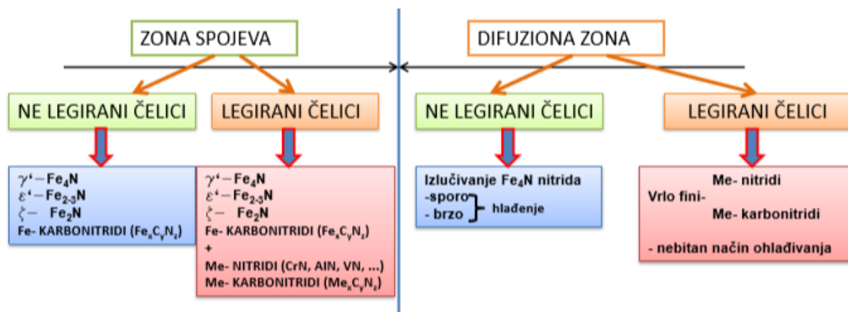
Slika 11. Sastav nitiranog sloja [13]
