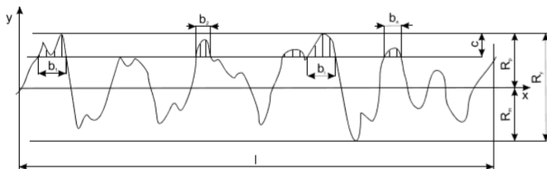
Slika 22. Najveća visina profila, R_y , najveća visina izbočine, R_p , najveća dubina izbočine, R_m [8]
