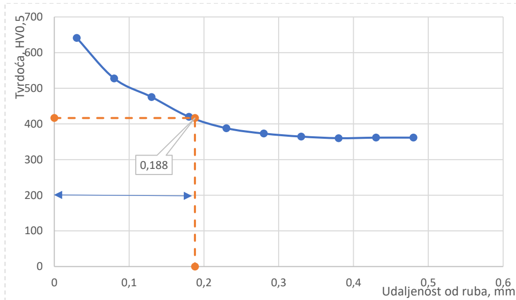
Slika 42. . Efektivna dubina nitriranja prstena nitriranog u plinu
