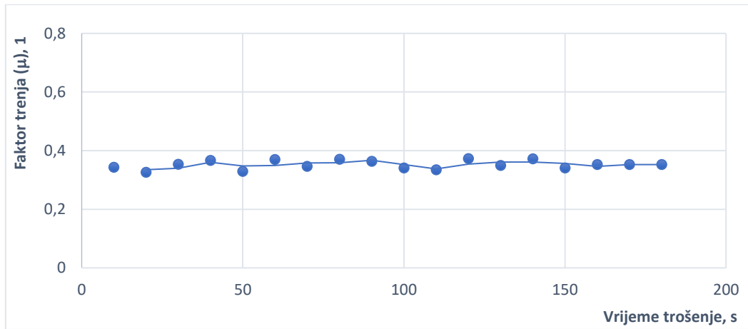
Slika 34. Faktor trenja za prsten nitriran u plinu
