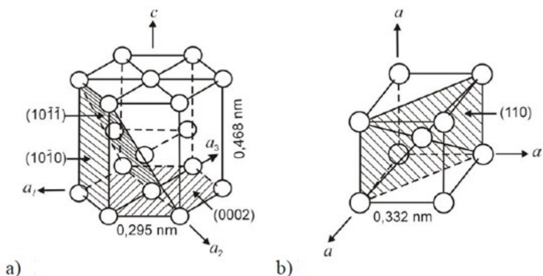
Slika 3. Prikaz alotropskih modifikacija titanija. (a) Heksagonska rešetka (HCP). (b) Kubična volumno centrirana rešetka (BCC)[5]
