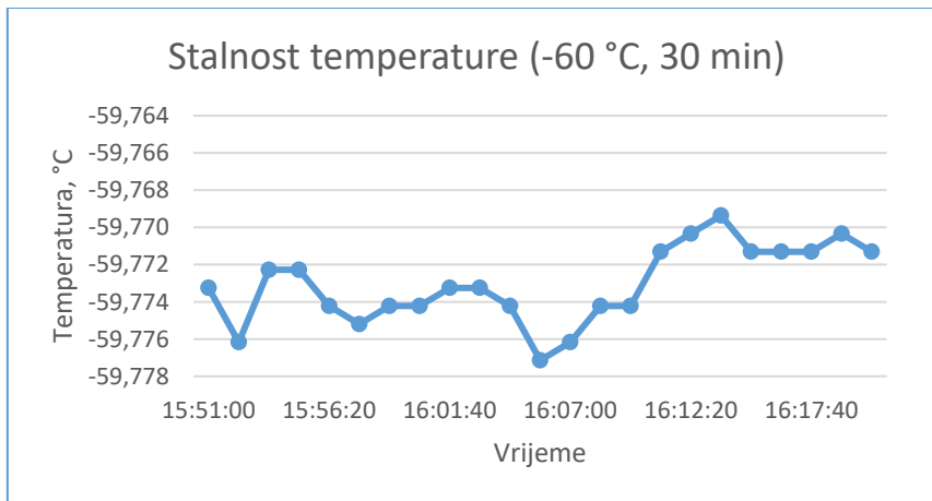
Slika 14. 30 minutna stalnost temperature pri -60 °C
