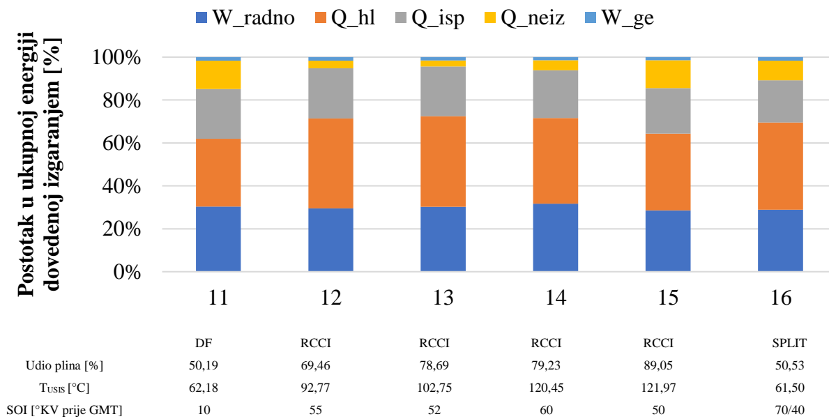
Slika 31. Postotna razdioba dovedene topline od 11. do 16. radne točke
