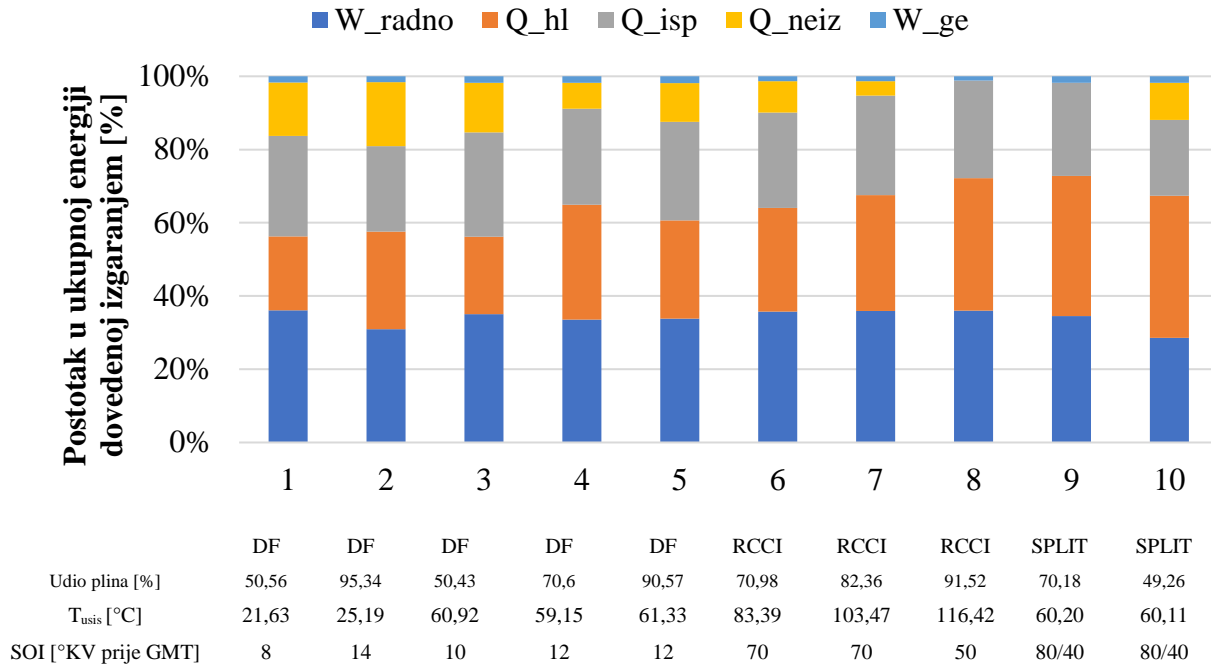
Slika 30. Postotna razdioba dovedene topline od 1. do 10. radne točke
