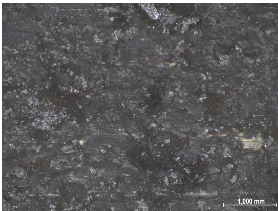
Slika 82. Snimak tragova trošenja kočione obloge 1 pri povećanju od 25x
