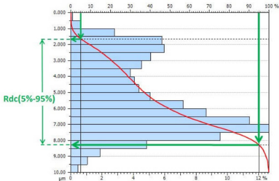
Slika 24. R_{dc} iznosi 6,5 \mu\text{m} za udio 5%-95% [13]
