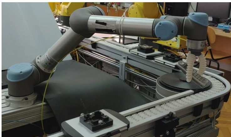
Slika 42. Prenošenje telefona pomoću meke prihvatnice
