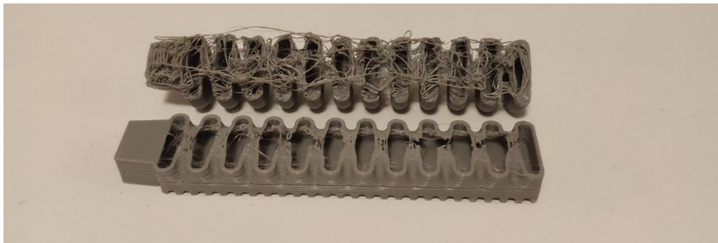
Slika 36. Greška u printanju nastala nepovezivanjem slojeva
