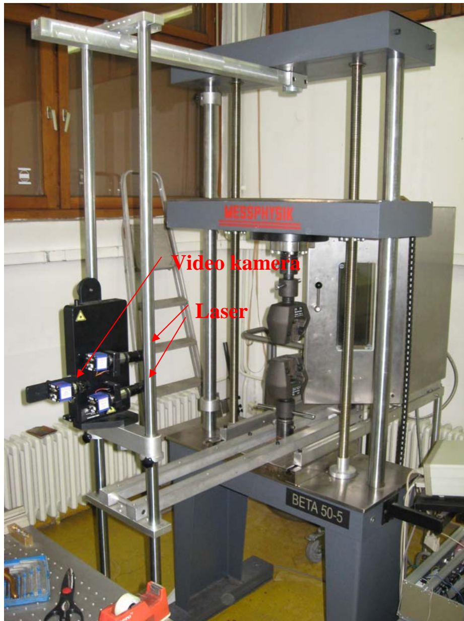
Slika 4.7. Postavljeni videoekstenzometar
