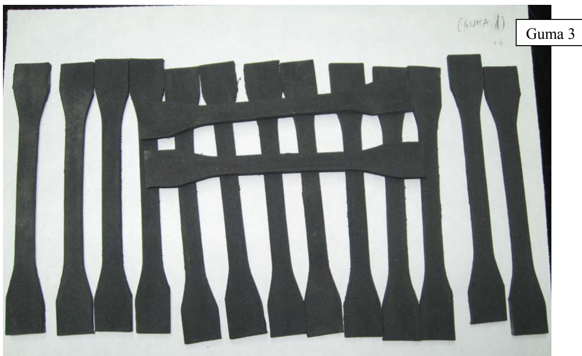
Slika 4.3. Pripremljene epruvete
