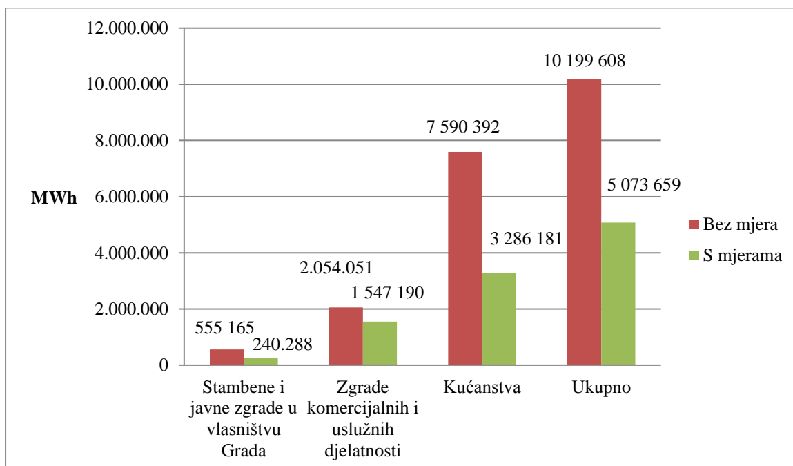
Slika 1. Usporedba potrošnje energije bez mjera i s mjerama za zgradarstvo Grada Zagreba
