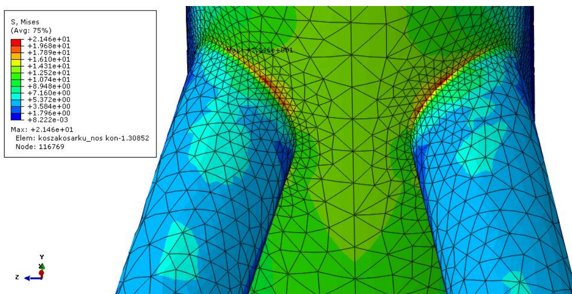
Slika 40. Detalj A - najveće naprezanje prema von Misesu na nosivoj konstrukciji u MPa
