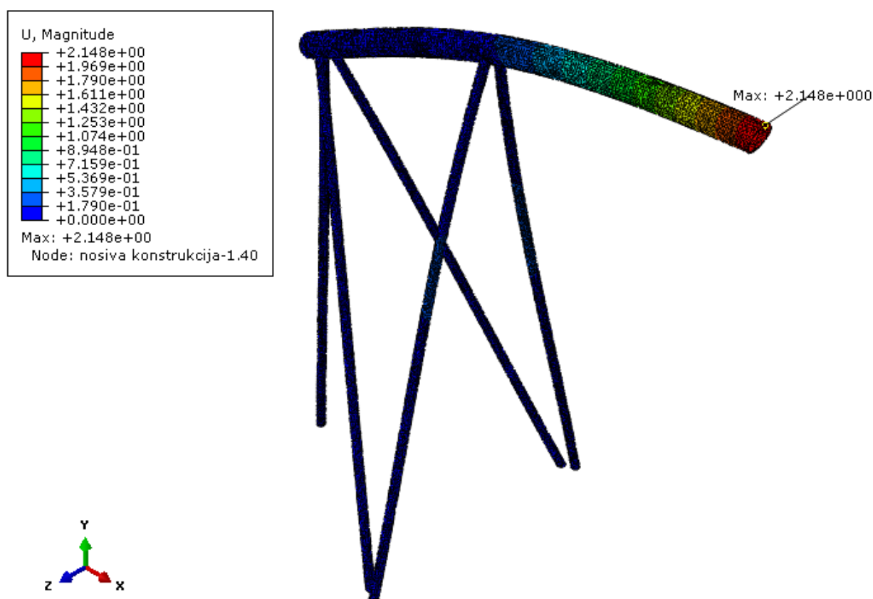
Slika 49. Pomaci u nosivoj konstrukciji u mm
