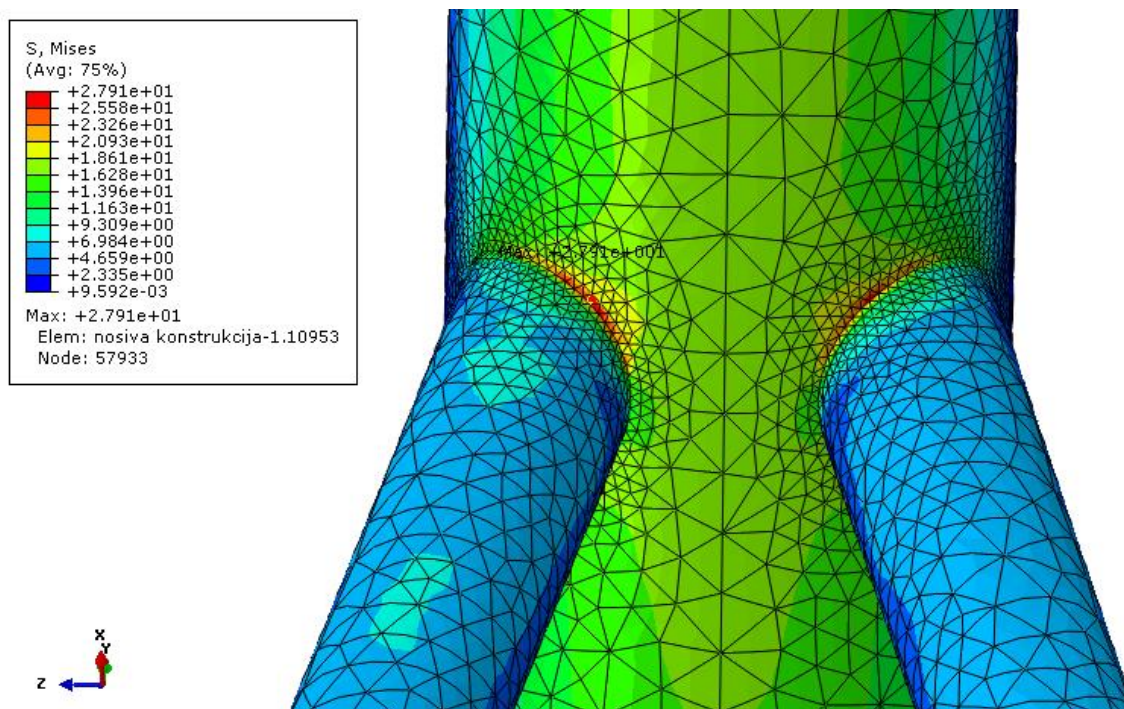
Slika 48. Prikaz maksimalnog napreznja u nosivoj konstrukciji prema Von Mises-u u Mpa
