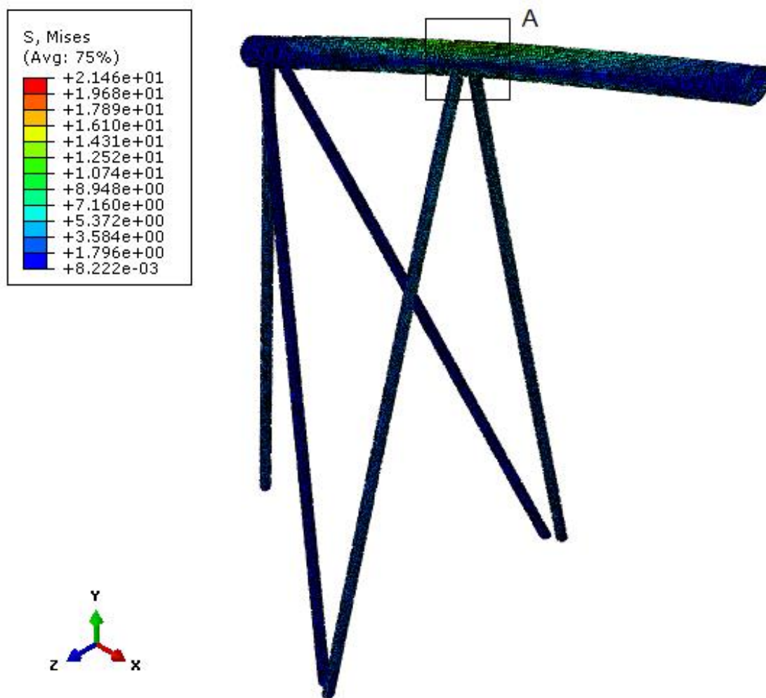
Slika 39. Naprezanje nosive konstrukcije prema Von Mises-u u MPa
