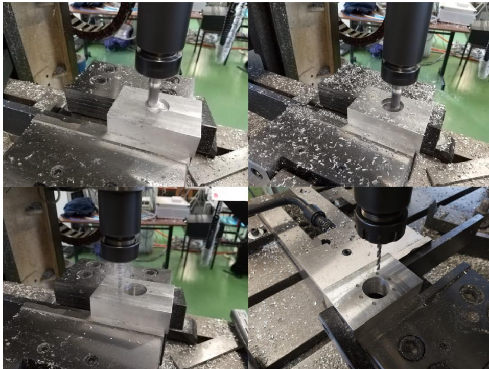
Slika 49. Izrada kućišta matice
