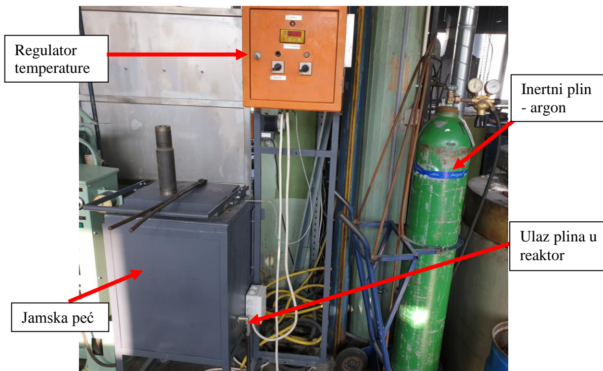
Slika 11. Jamska peć
