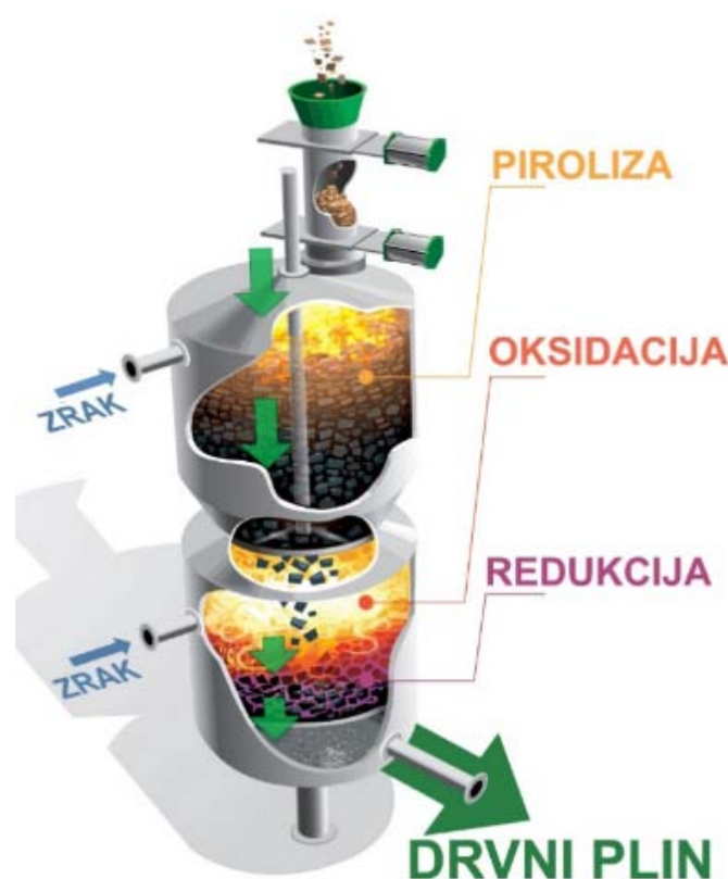
Slika 17. Faze rasplinjavanja [23]
