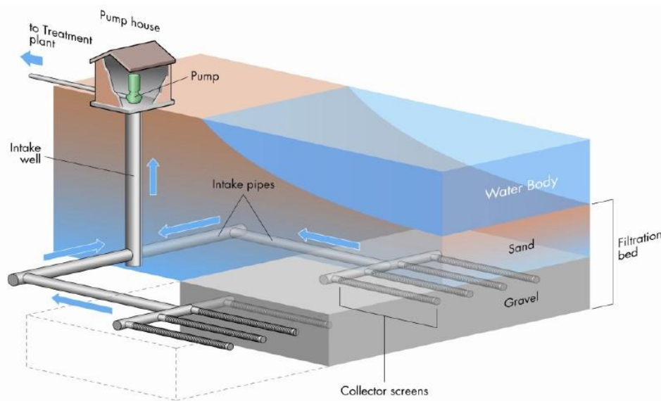
Slika 2.11 Zahvat morske vode infiltracijom kroz morsko dno [17]
