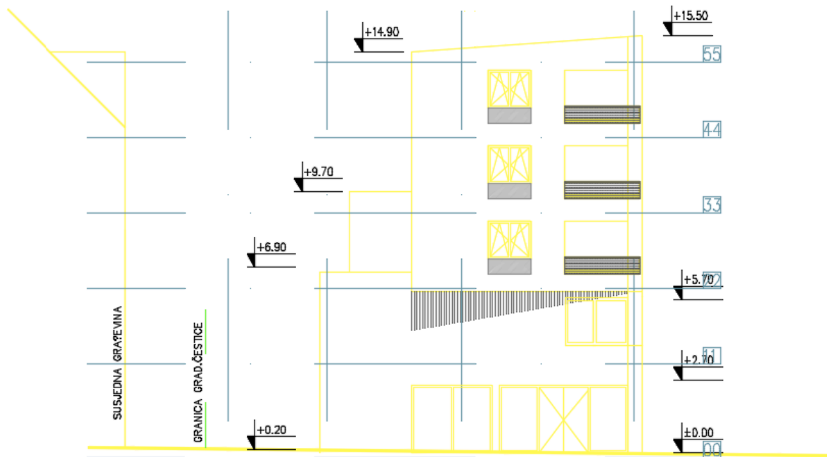
Slika 16. Pročelje zapad
