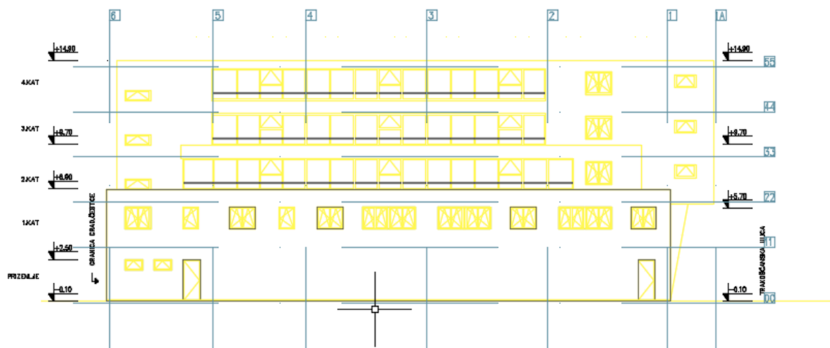
Slika 14. Pročelje sjever
