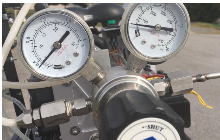
Slika 43. Regulator tlaka
