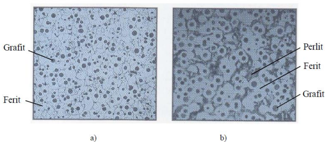
Slika 1. Mikrostruktura nodularnog lijeva: a) feritna matrica b) perlitno-feritna matrica [1]
