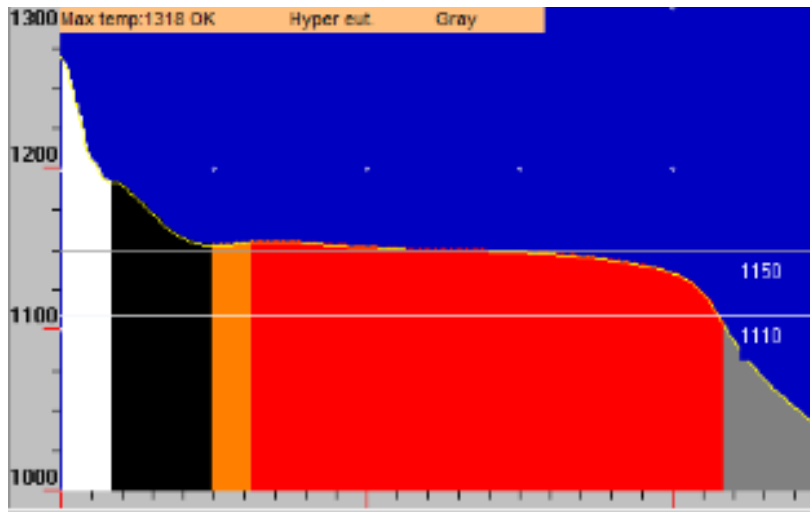
Slika 30. Krivulja hlađenja nodularnog lijeva
