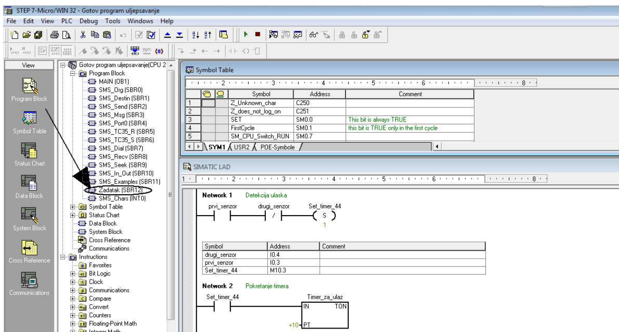
Slika 6.1 Podprogram „Zadatak“
