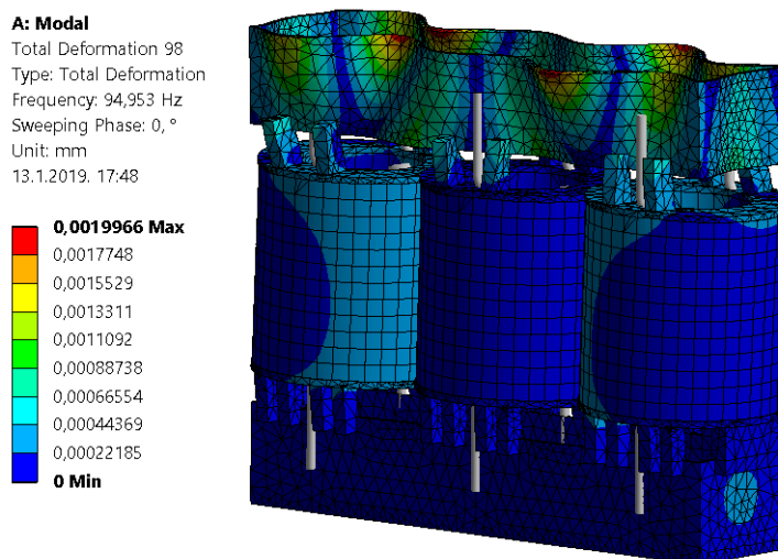
Slika 8.14. Vlastita forma vibriranja (94,953 Hz)
