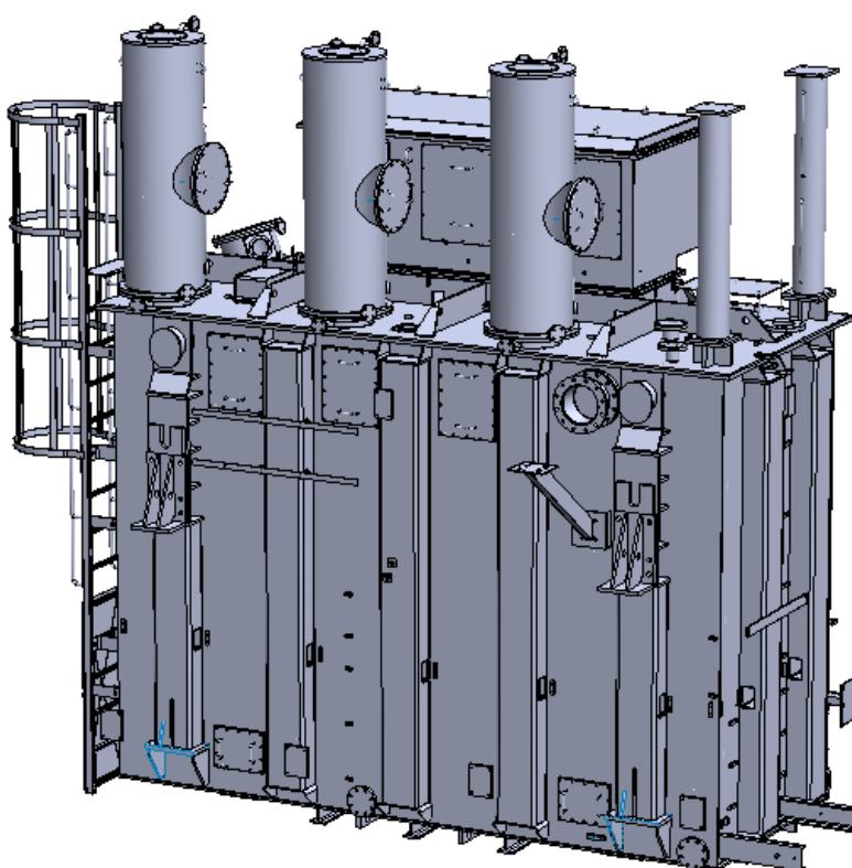
Slika 5.1. Kućište transformatora, [10]
