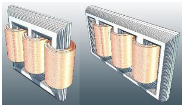
Slika 2.9. Trofazne jezgre, [7]
