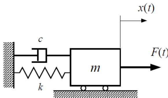
Slika 3.3. Sustav sa jednim stupnjem slobode gibanja, [2]
