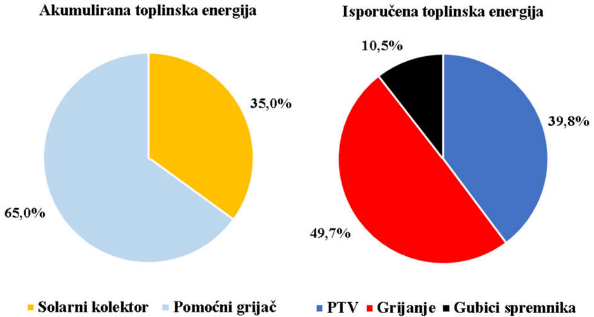
Slika 38. Udjeli akumulirane i isporučene toplinske energije iz spremnika na godišnjoj razini za zgradu s Q_{H,nd} = 20 \text{ kWh/m}^2\text{a} – satna metoda sa stratifikacijom temperature u spremniku
