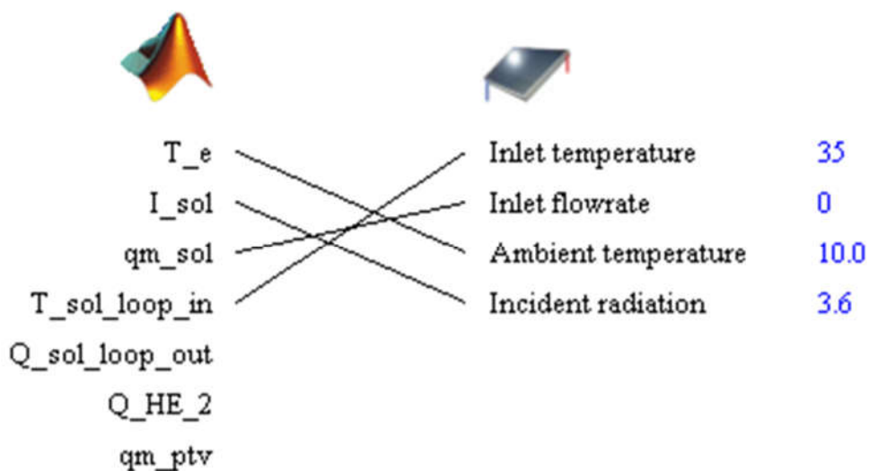
Slika 2. Povezivanje izlaznih i ulaznih varijabli komponenta unutar programa Simulation Studio
