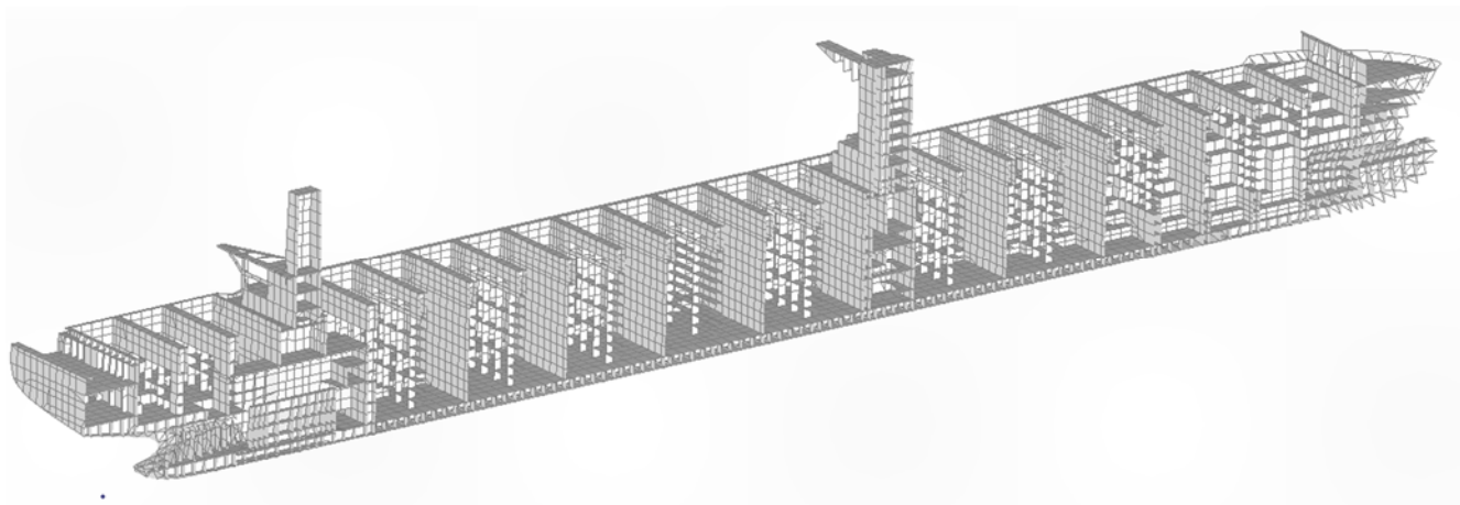
Slika 24. Uzdužni presjek broda
