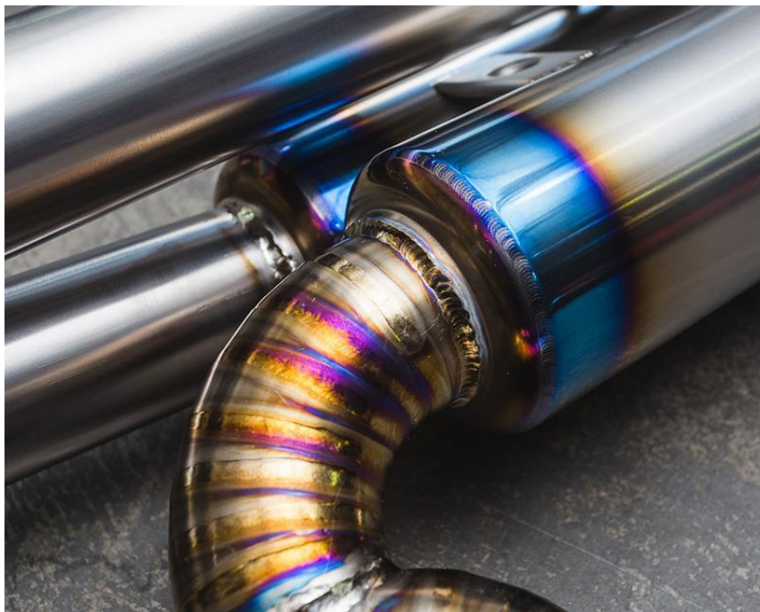
Slika 4.1. Zavarivanje titanijevog ispušnog sustava [27]
