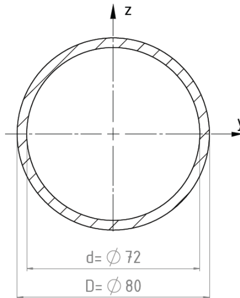
Slika 59. Presjek vertikalnog nosača
