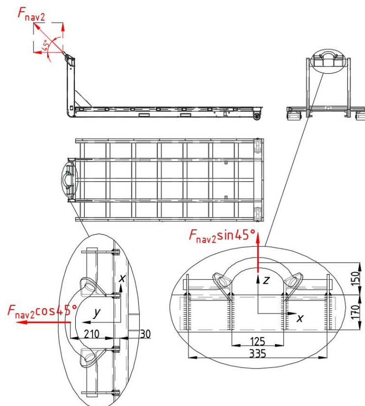
Slika 3.67. Shema opterećenja i presjek zavara prihvata kuke navlakača
