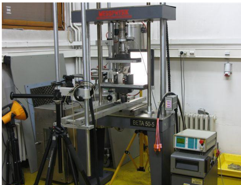
Slika 26. Kidalica MESSPHYSIK BETA 50-5 u laboratoriju za eksperimentalnu mehaniku
