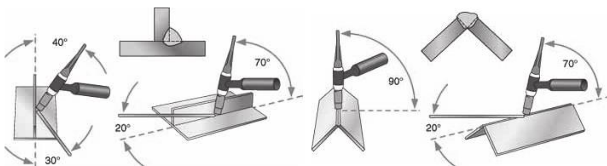
Slika 16. Izvođenje kutnog (lijevo) i rubnog (desno) spoja [15]
