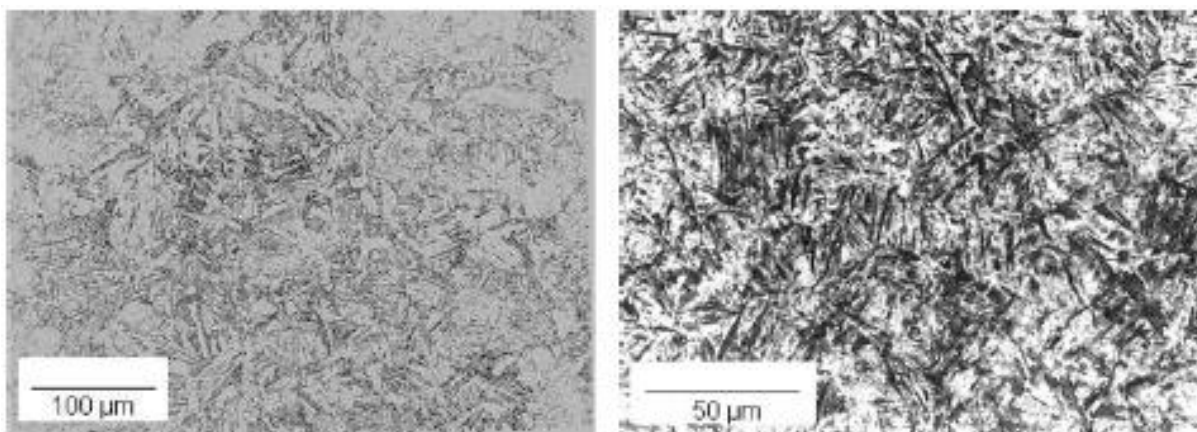
Slika 6. Mikrostruktura martenzitnog nehrđajućeg čelika [1]
