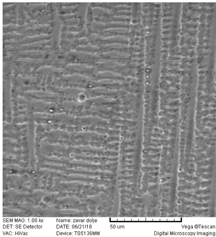
Slika 46. Zavar dolje uzorka uz povećanje 1000 x
