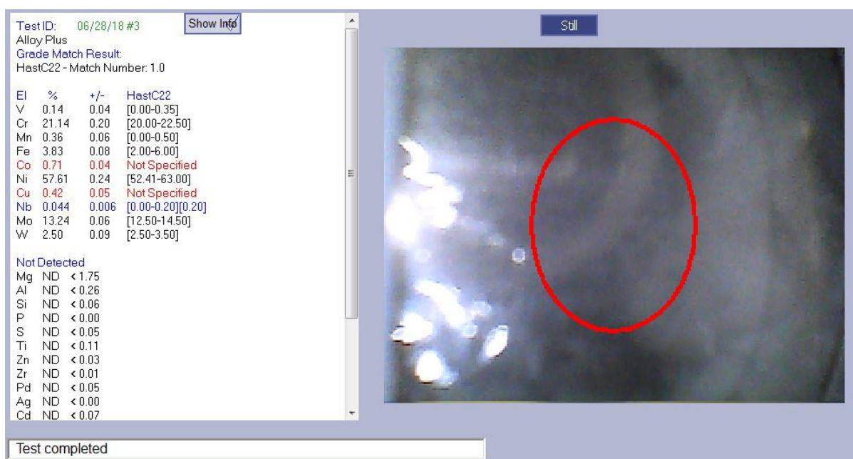
Slika 55. Kemijski sastav osnovnog materijala
