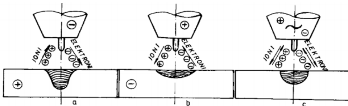
Slika 8. Oblici zavara u ovisnosti o vrsti struje:
