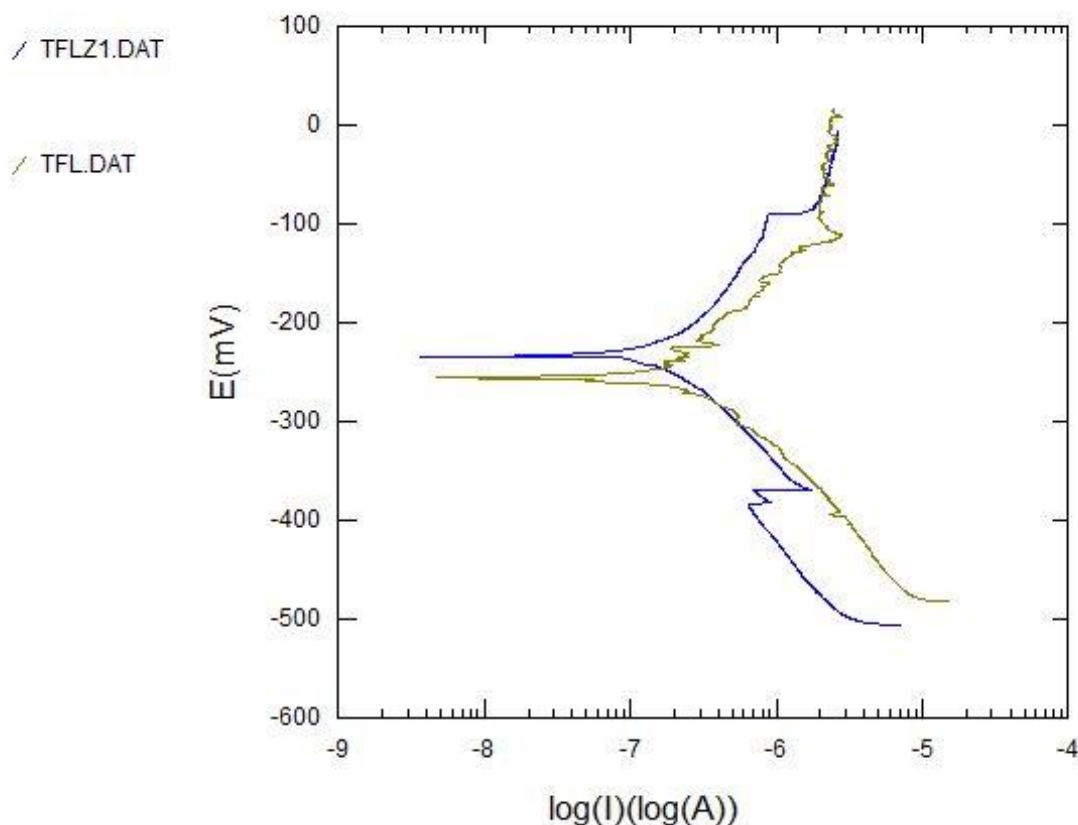
Slika 52. Preklop krivulja osnovnog materijala i metala zavara kod Tafelove metode
