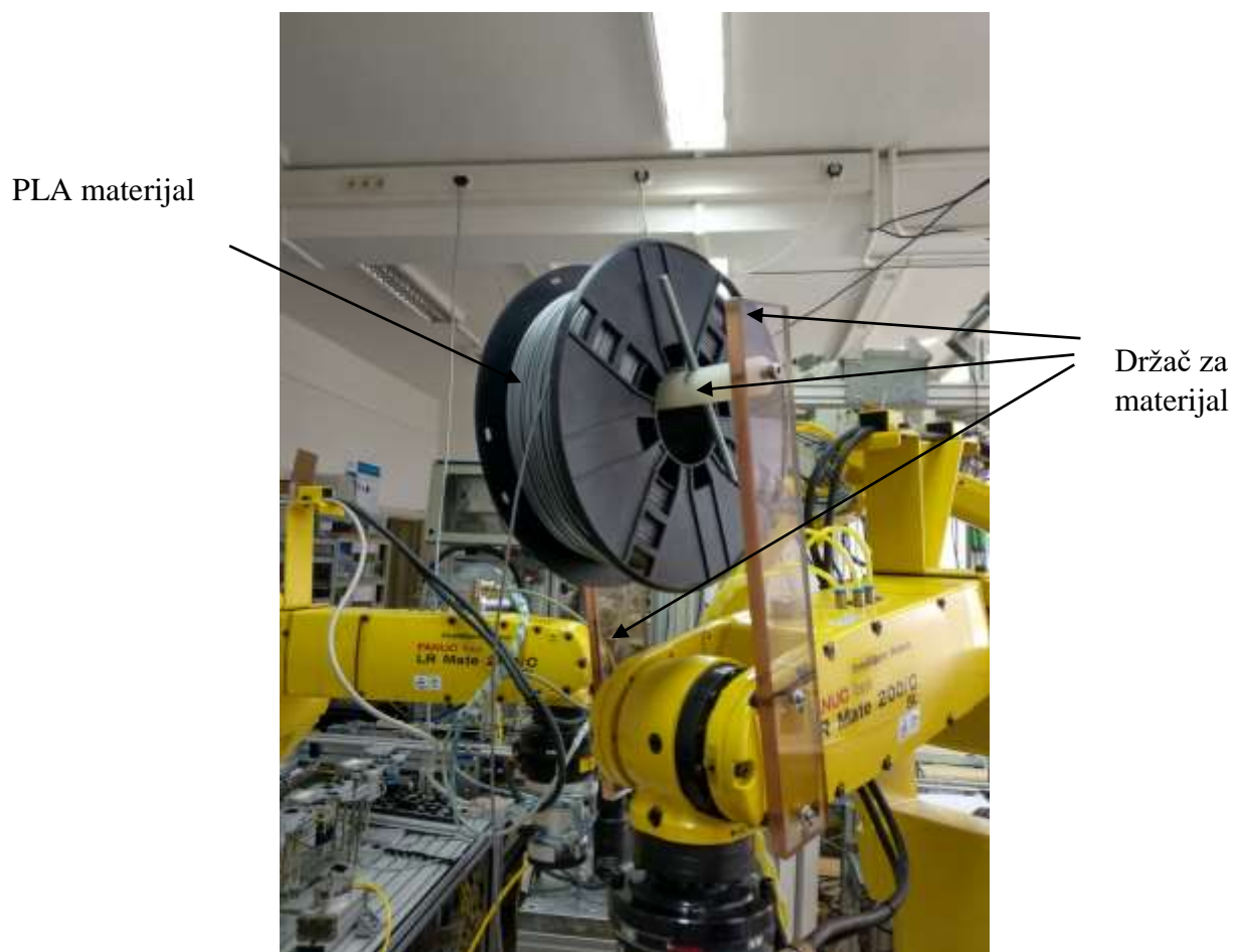
Slika 8. Držač za materijal
