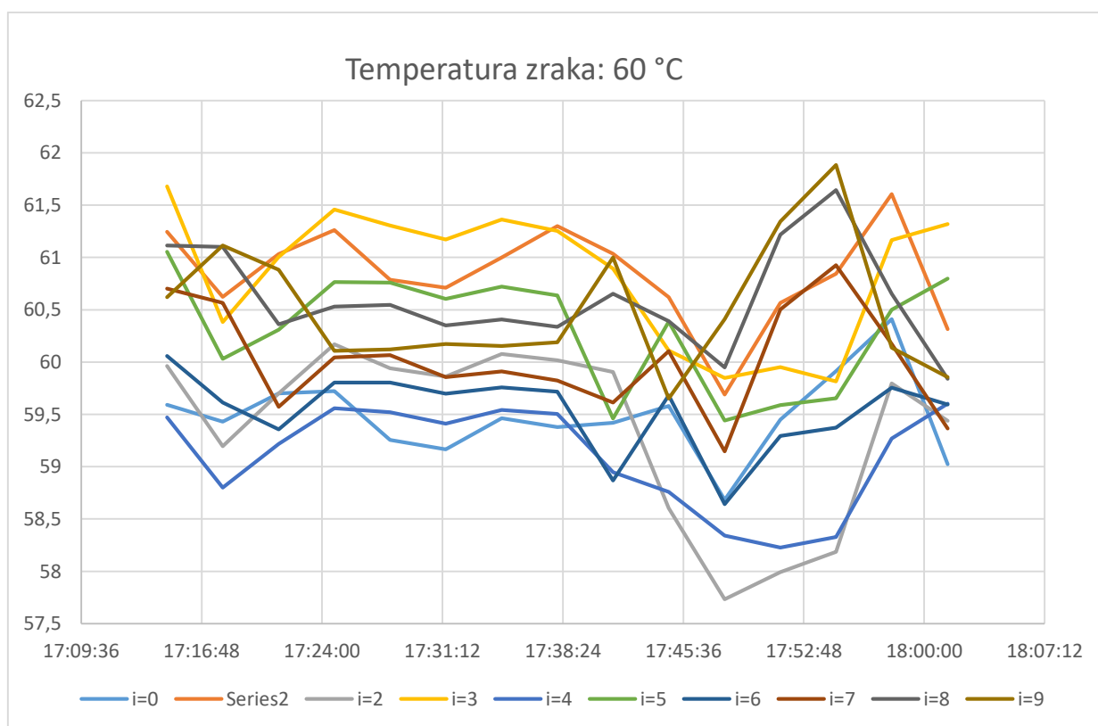
Slika 18. Prikaz temperatura u komori tokom mjerenja u svim mjernim točkama (T = 60 °C)
