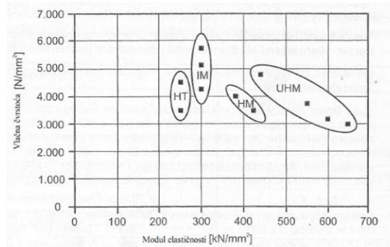
Slika 2.8. Podjela ugljičnih vlakana (7)
