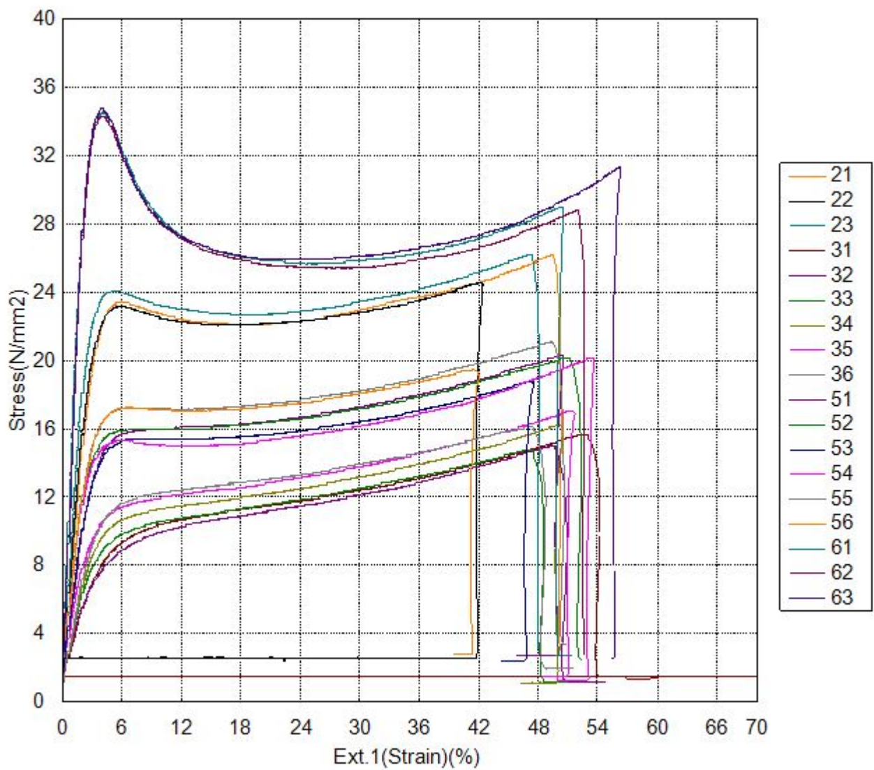
Slika 4.5: Naprežanje - deformacija grafovi za testirane epruvete Grafovi naprežanje - deformacija dobiveni programom integriranim u kidalici
