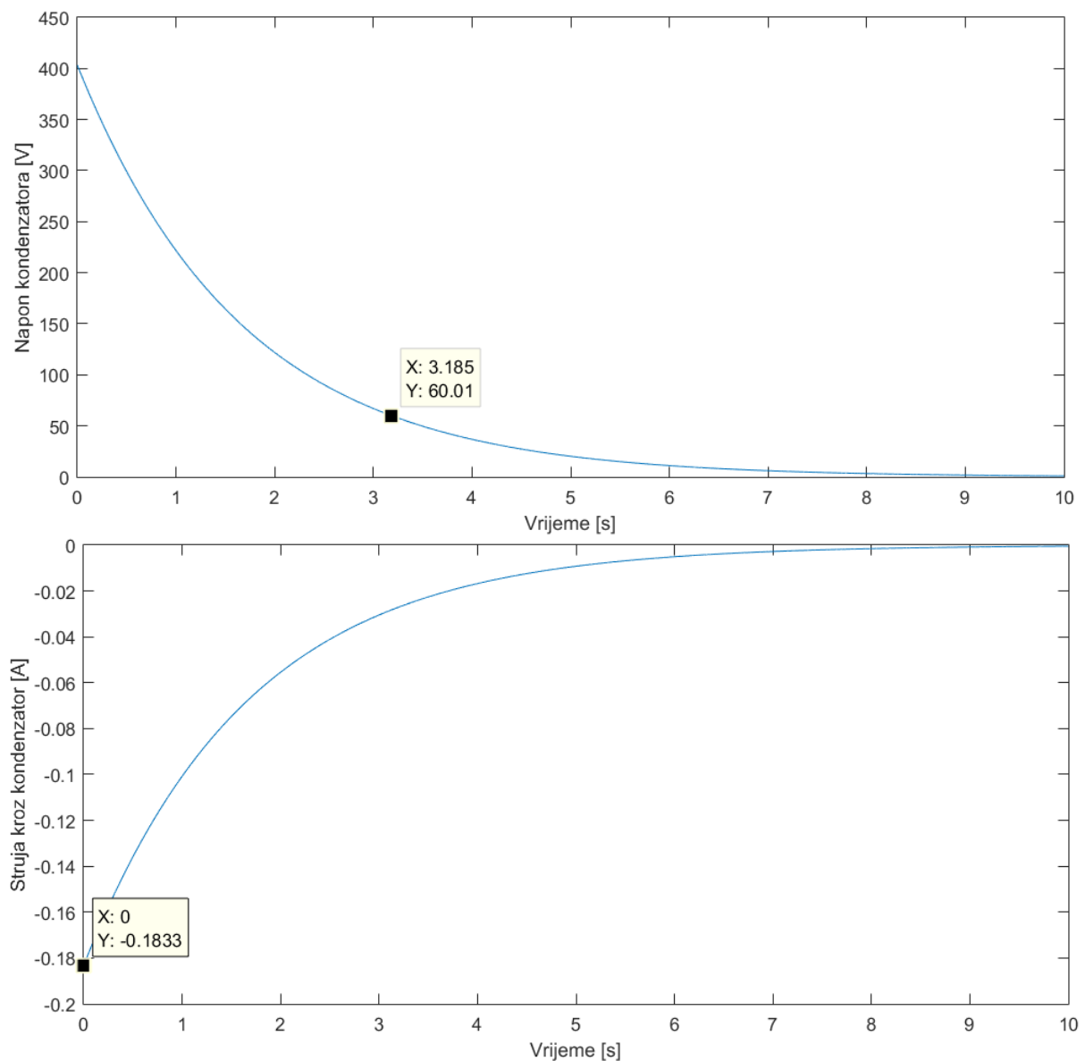
Slika 29. Pražnjenje kondenzatora preko otpora od 2,2 k \Omega
