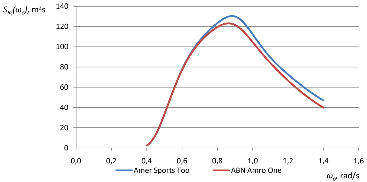
Dijagram 13. Spektri odziva za \beta_3
