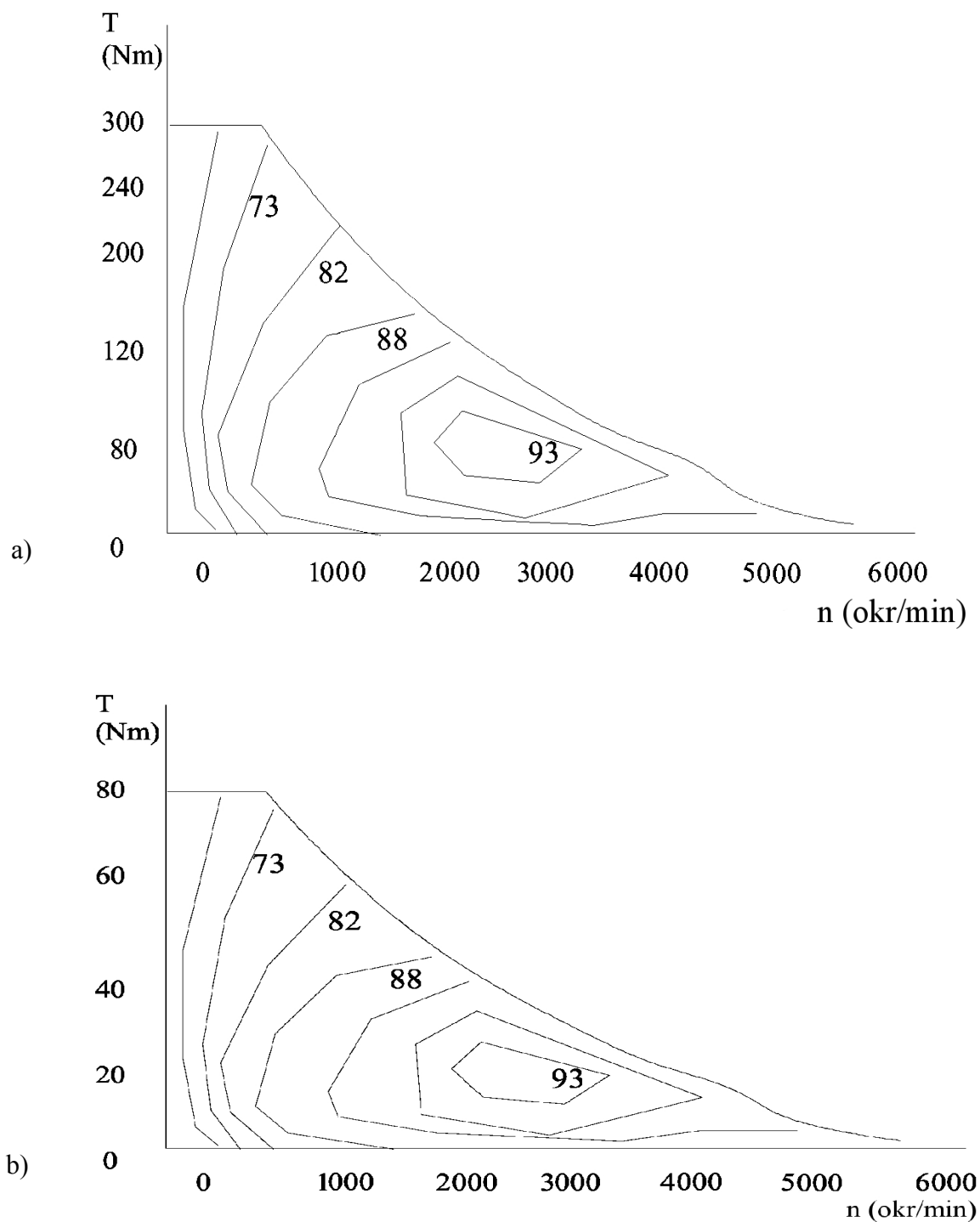
Slika 2.11: Primjer momentnih karakteristika za elektromotore kod hibridnog vozila Toyota Prius (a) za traksijski elektromotor (M/G2), (b) za generator (M/G1) [6]
