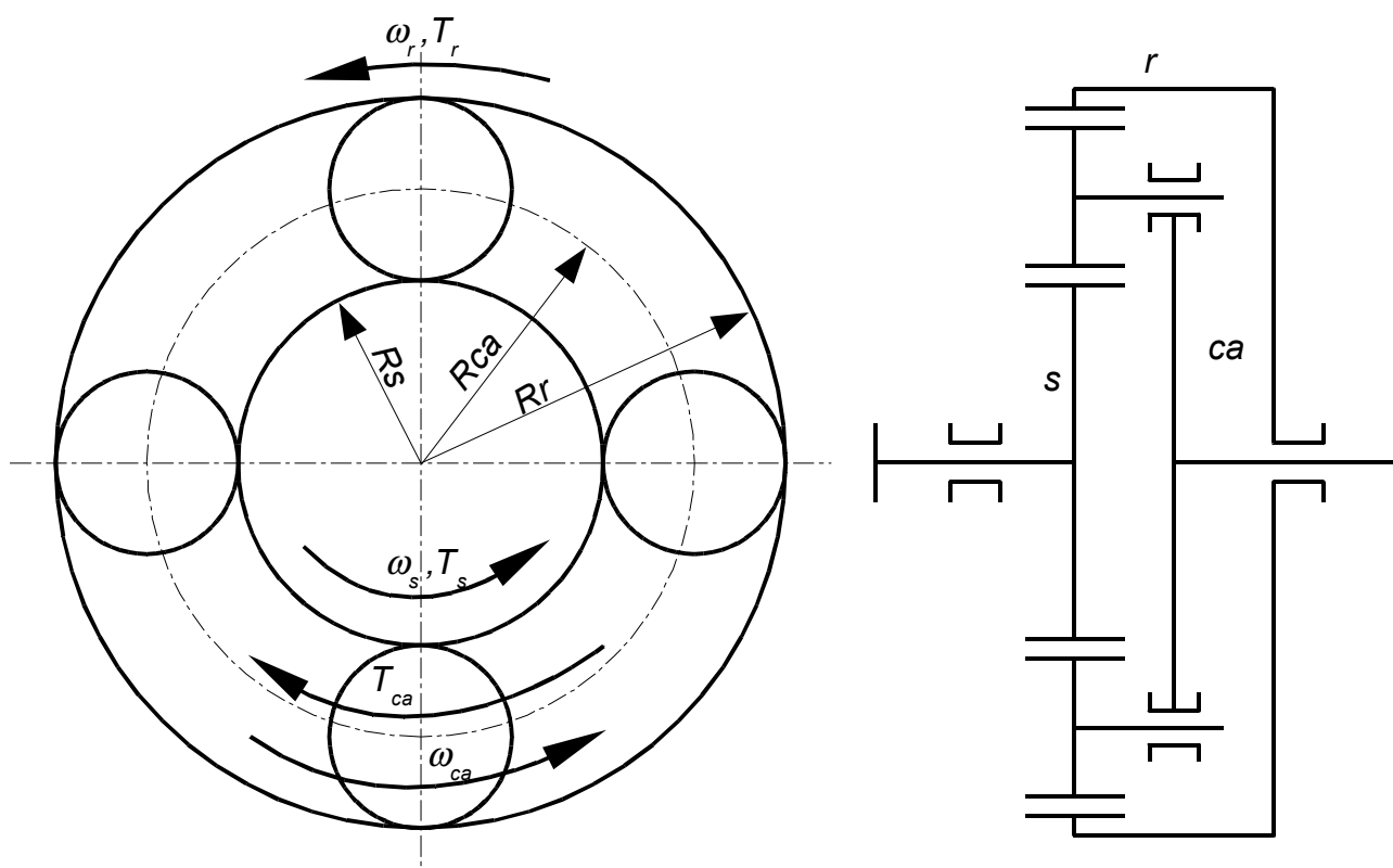
Slika 3.7: Shema planetarnog prijenosnika
