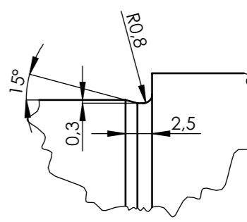
Detalj D (M 2:1)
