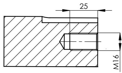
C-C (M 1 : 1)
