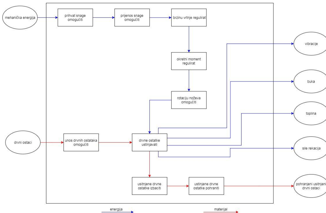
Slika 10. Funkcijska dekompozicija
