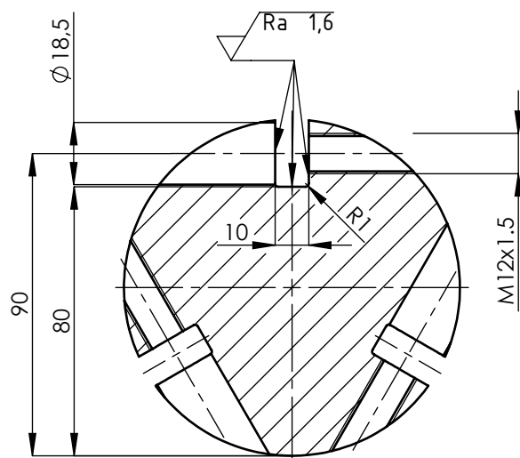
A-A (M 1:2)
