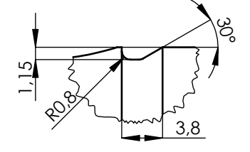
Detalj F (M 2:1)
