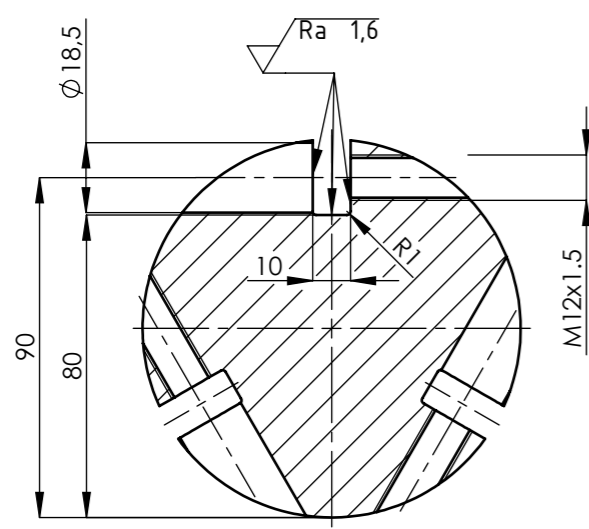
A-A (M 1:2)
