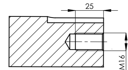
C-C (M 1:1)
