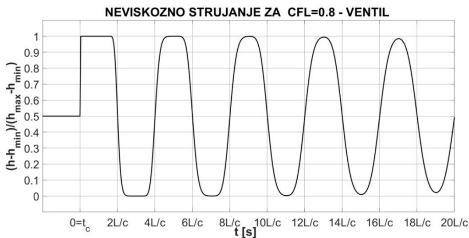
Slika 44 – Promjena piezometričke visine na mjestu ventila pri neviskoznom strujanju fluida za CFL = 0,8
