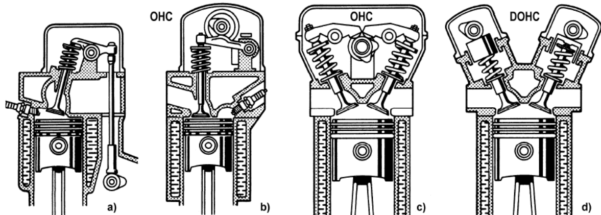
Slika 2. Viseći ventili: a) bregasto vratilo u bloku; b), c) i d) bregasto vratilo u glavi [1] Razvodni mehanizam prema položaju bregaste osovine dijelimo na:
