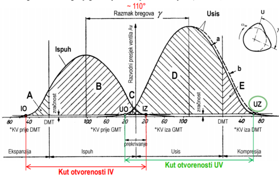
Slika 10. Razvodni dijagram 4T motora [1]
