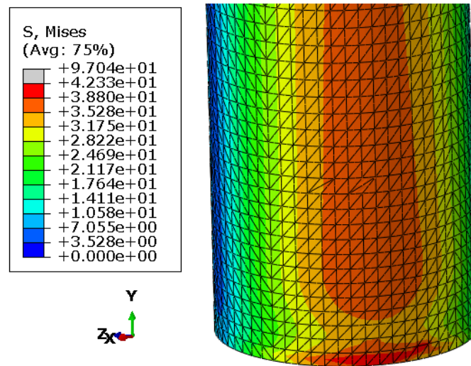
Slika 36. Raspodjela naprezanja u MPa na mjestu uklještenja s ograničenjem na 42,33 MPa
