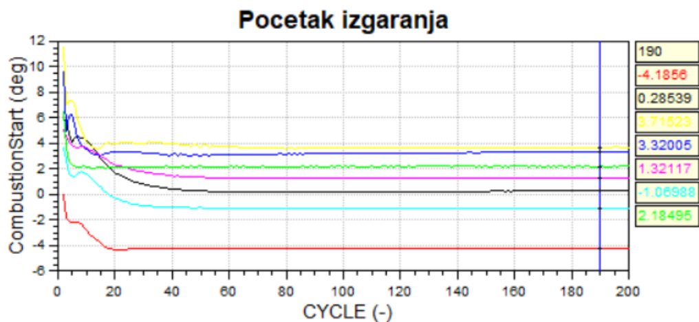
Slika 14. Dijagram konvergencije traženog početka izgaranja
