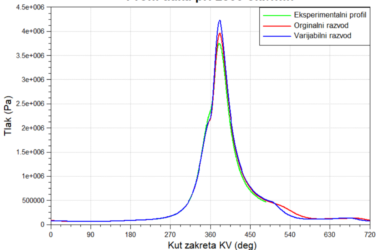
Slika 27. Profil tlaka u cilindru pri 2500 okretaja u minuti
