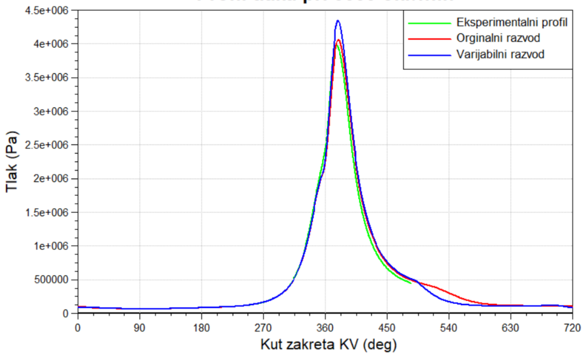
Slika 28. Profil tlaka u cilindru pri 3000 okretaja u minuti
