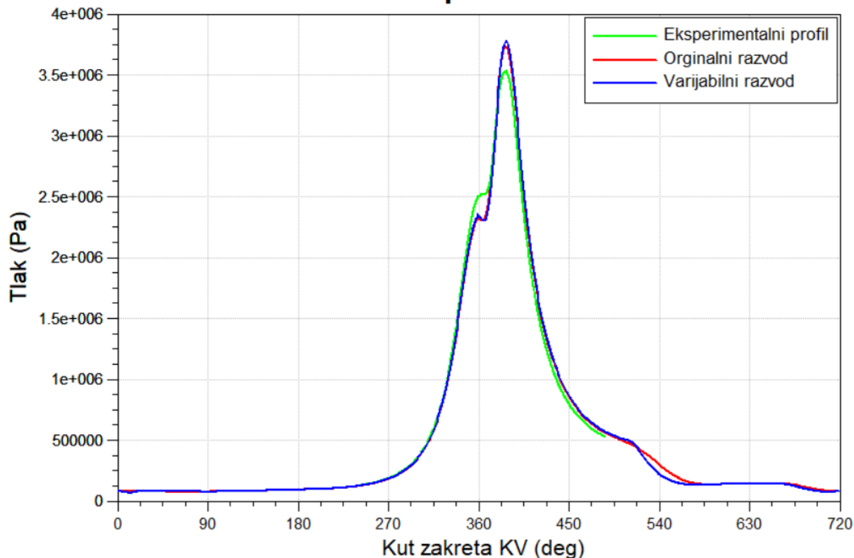
Slika 25. Profil tlaka u cilindru pri 2000 okretaja u minuti
