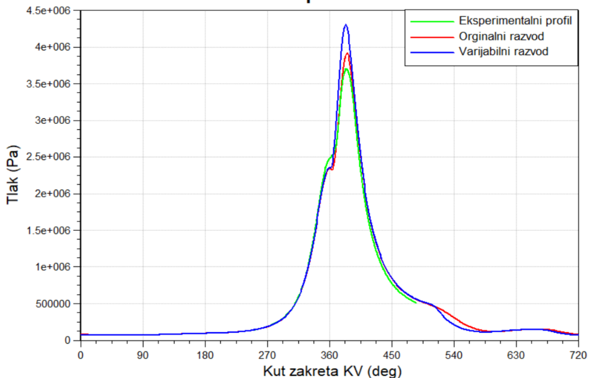
Slika 26. Profil tlaka u cilindru pri 2200 okretaja u minuti
