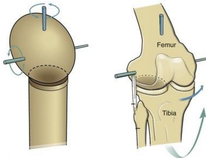
Slika 12. Zglob koljena [15]
