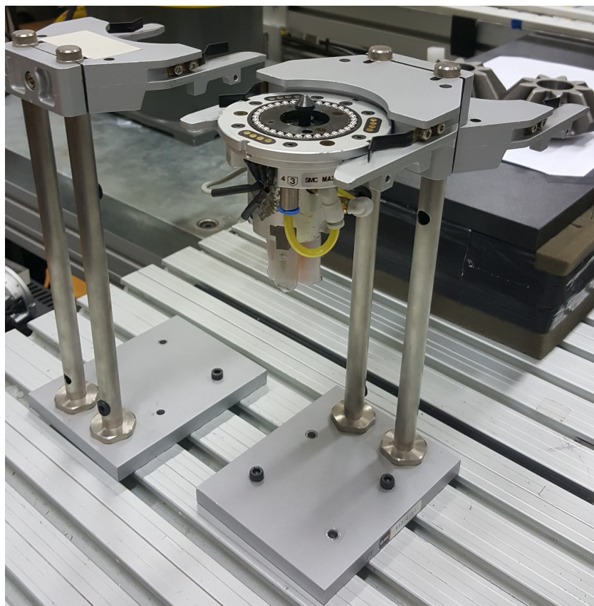
Slika 34. Prikaz troprosnje hvataljke
