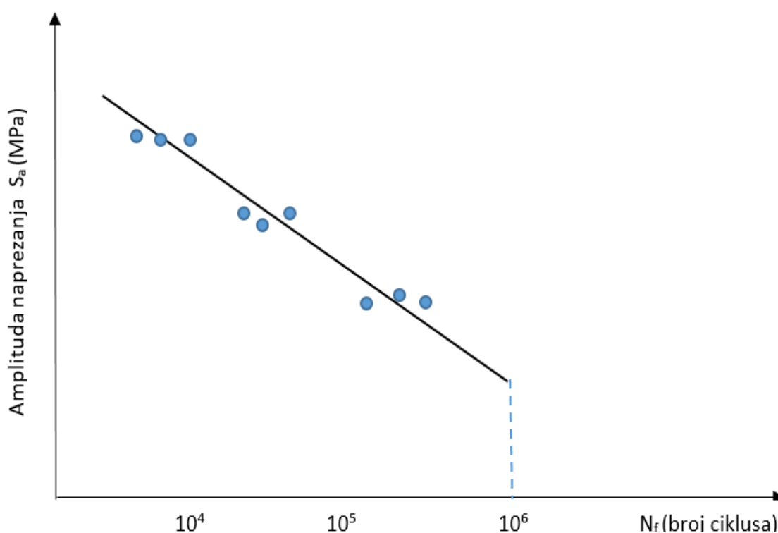
Slika 15 Određivanje konačnog dijela S-N dijagrama
